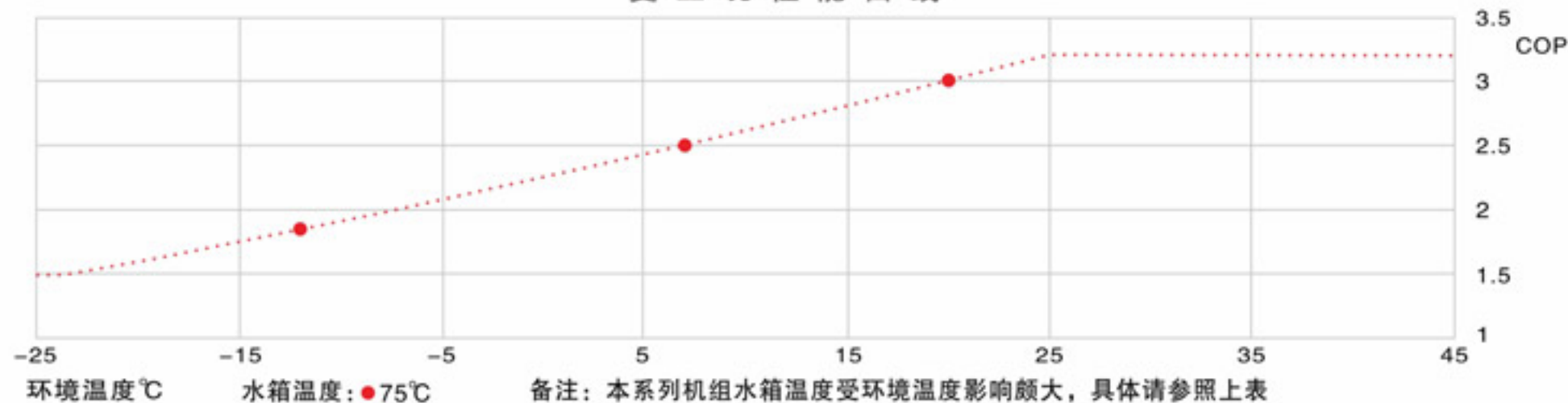
变工况性能曲线
